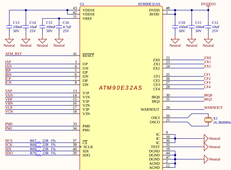
ENERGY METER IC
